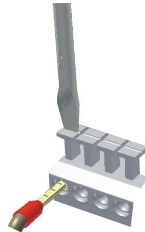
Abb. 8.4 Einbringen der Kabel in das Verbindungsstück
