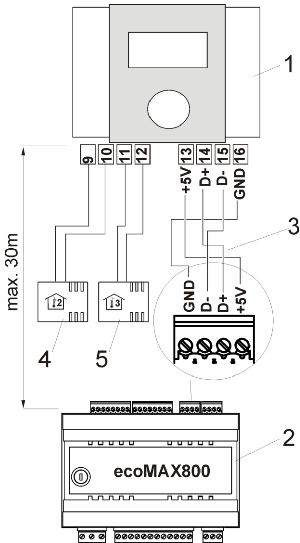
Abb. 8.3 Schema des elektrischen Anschlusses; wobei: 1 - Zimmerpanel ecoSTER200, 2 - Regler ecoMAX800, 3 - Verbindungskabel, 4 - Temperaturfühler Thermostat 2 Typ CT7, 5 - Temperaturfühler Thermostat 3 Typ CT7.
