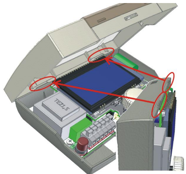
Abb. 8.5 Schließen des Gehäuses, Schritt 1 (Zeichnung zur Ansicht)
