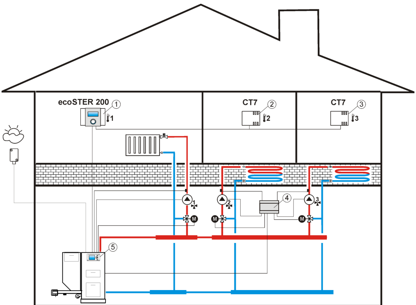
Abb. 8.7 2 Schema - Zusammenarbeit ecoSTER - ecoMAX800, wobei: 1 - ecoSTER200, 2- Zimmerfühler Thermostat 2 Typ CT7, 3 - Zimmerfühler Thermostat 3 Typ CT7, 4- Modul MX.01 (erweitert das System um 2 Heizkreise), 5 - Regler ecoMAX800.
