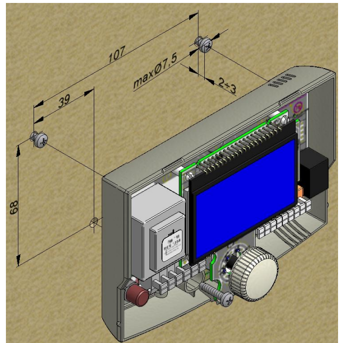
Abb. 8.2 Anbringen des Reglers an der Wand (Zeichnung zur Ansicht)
